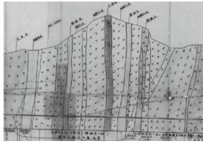
仙山線 仙山隧道地質図
